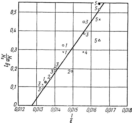
Р и с. 12.3. Зависимость \lg \frac{sK}{wK} от \frac{1}{\epsilon} .
