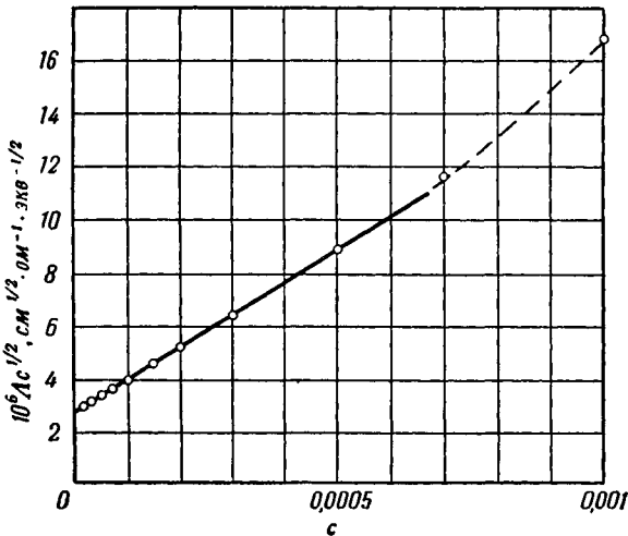
Рис. 14.4. График зависимости \Lambda\sqrt{c} от c для азотно-кислого тетраизоамиламмония в смеси диоксан—вода, имеющей диэлектрическую постоянную 2,56.
