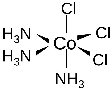
fac -[CoCl 3 (NH 3 ) 3 ] гран -[CoCl 3 (NH 3 ) 3 ]
