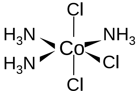
mer -[CoCl 3 (NH 3 ) 3 ] ос -[CoCl 3 (NH 3 ) 3 ]
