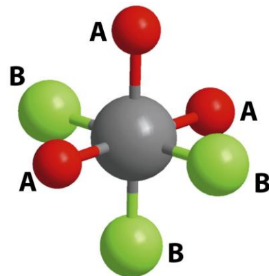
mer -[CoCl 3 (NH 3 ) 3 ] ос -[CoCl 3 (NH 3 ) 3 ]
