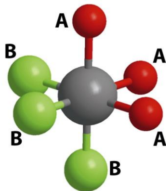
fac -[CoCl 3 (NH 3 ) 3 ] гран -[CoCl 3 (NH 3 ) 3 ]
