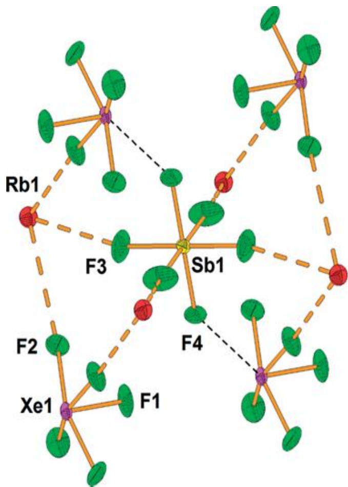
\text{Rb}[\text{XeF}_5](\text{SbF}_6)_2
