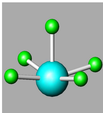
\text{XeF}_5^+
